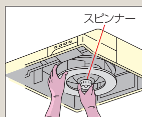
スピナーを「ユルム」の方向に回し、ターボファンを手で支えながらははずす。
