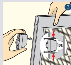
3 戸車のネジを締めて固定する。
