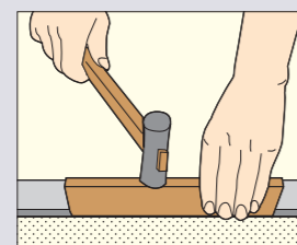
棒状ガスケットは手ではめした後、木片と金づちではめ込む。
