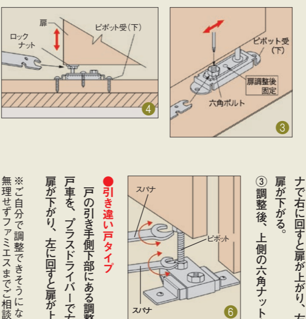
扉を上げる。扉を下げる。
