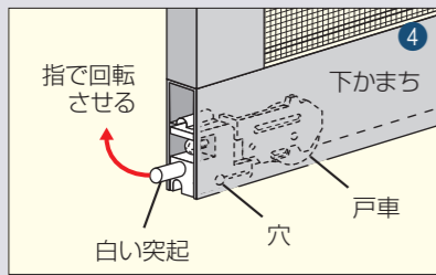
4 網戸を下枠の端に押し込み、突起を指で押し上げて90度回転させる。
