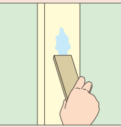
② ①へこんだ部分にヘラまたは指で白い木工用パテを塗り込む。
