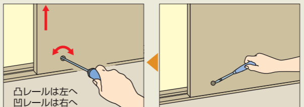
凸レールは左へ、凹レールは右へ回すと引き戸が持ち上がる。マイナスイドライバーで引き戸下にあるキャップをはずす。
