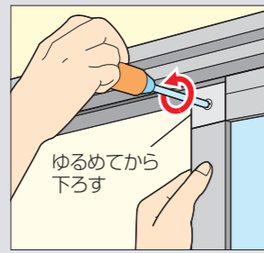
網戸の室外側にネジがあるタイプ
