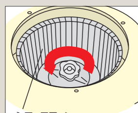
中央のつまみを「ユルム」の方向に回し、シロッコファン本体を手で押さえながらははずす。
