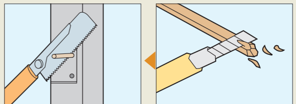
木工用接着剤でしっかり固定したら、余分な箸を切り落とす。ネジ穴の大きさに合わせて割り箸を細く削る。
