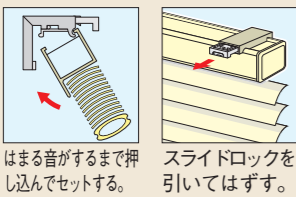
はまる音がするまで押し込んでセットする。スライドロックを引いてはずす。
