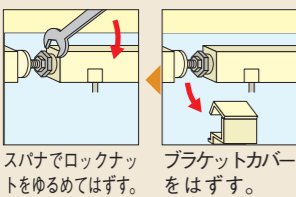
スパナでロックナットをゆるめず。ブラケットカバーをはずす。
