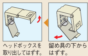
ヘッドボックスを取り出してはずす。留め具の下からははずす。
