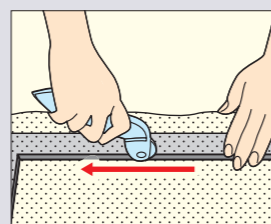
ゴム製ガスケットは各辺の中心から角に向けてはめ込む。
