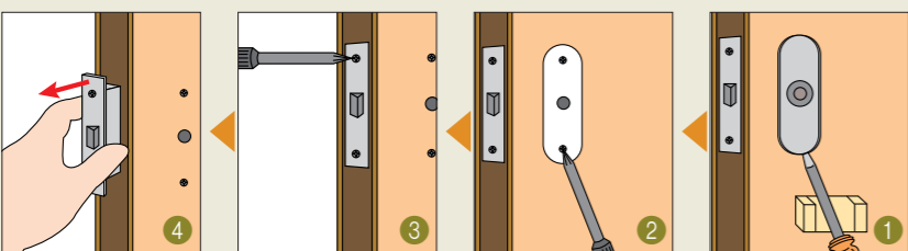
1 上の①～③の要領でハンドルを引き抜いた後、室外側の台座カバーをはずす。浮かしたカバーを90度回転させてから、2ヶ所のネジをしっかりと締める。 2 台座の2ヶ所のネジを抜き、台座そのものを取りはずす。 3 フロント板の2ヶ所のネジを抜き、フロント板をはずす。 4 本体を取り出した後、逆の手順で新しいハンドルを取り付ける。
