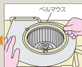
シロッコファンのベルマウスを取り付けネジ3ヶ所を手でははずし、ベルマウスをはずす。
